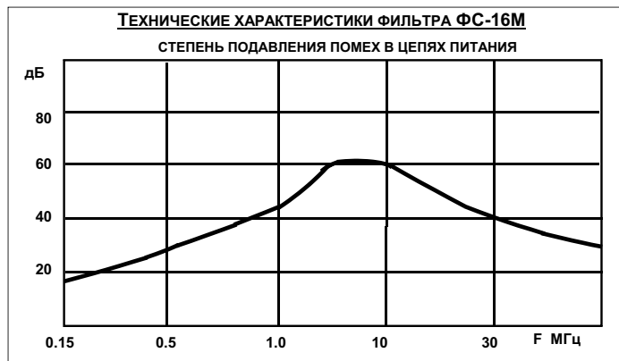
Рис.2. График АЧХ фильтра ФС-16М .
