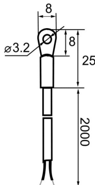
Габаритный размер датчика (заказывается отдельно)
